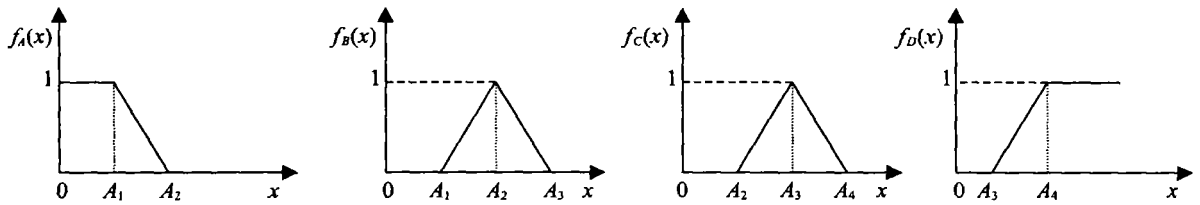
图2 交通安全评价灰类的白化权函数 Fig.2 Gray function of traffic safety evaluation
