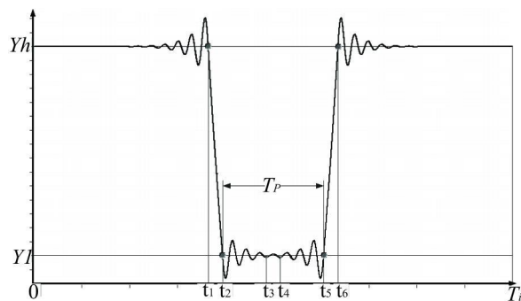
图 3 第 i 个脉冲的 y-t 图
