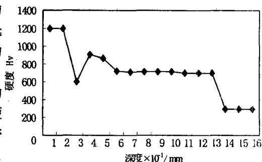
图4 激光合金化后典型的硬度曲线
