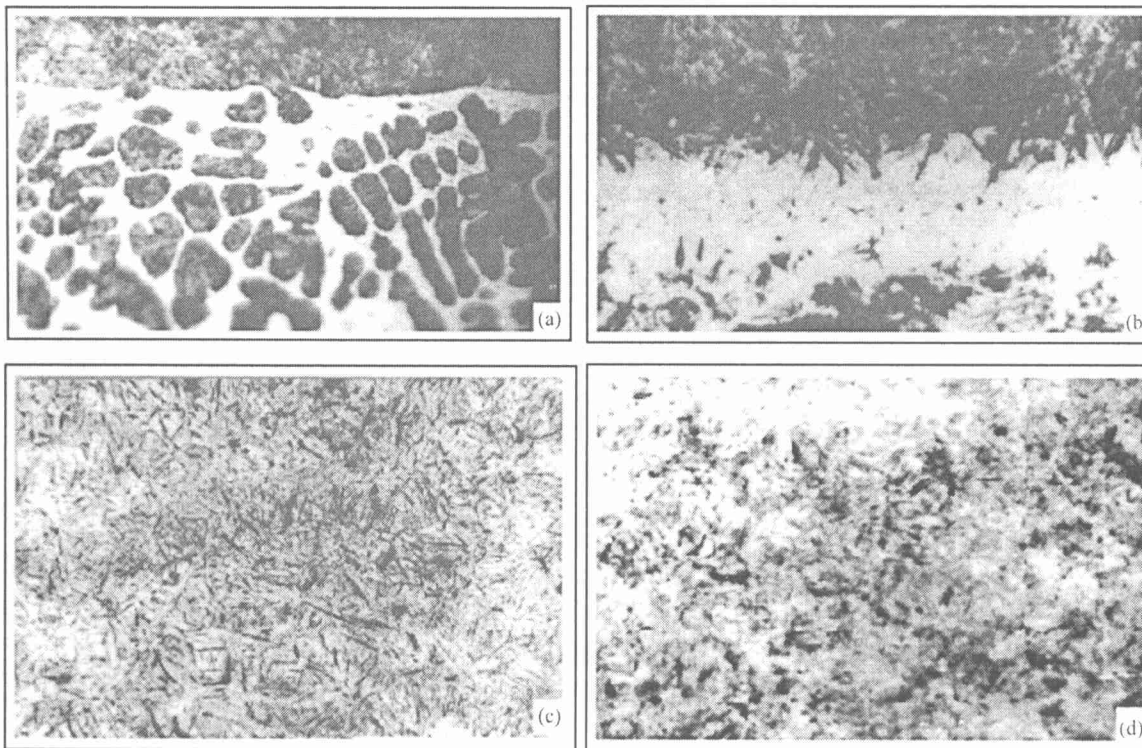
(a) 合金化区 (b) 过渡区 (c) 热影响区的针状马氏体 (d) 热影响区的隐晶马氏体
