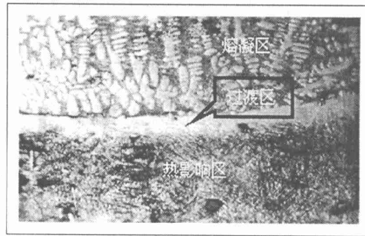
图 1 熔池截面形貌(100×)
