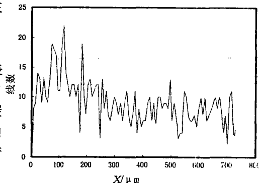
图3 深度方向上碳元素分布的线扫描分析结果
