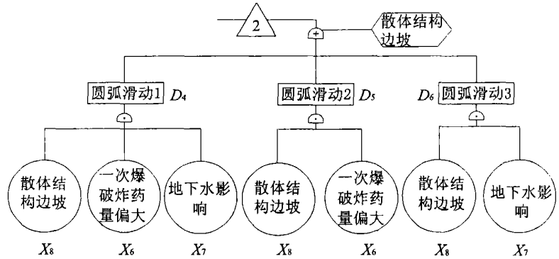
图3 圆弧滑动 Fig.3 Arc slippage
