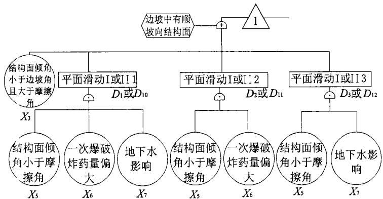
图2 平面滑动 I 或 II Fig.2 Plane slippage I or II
